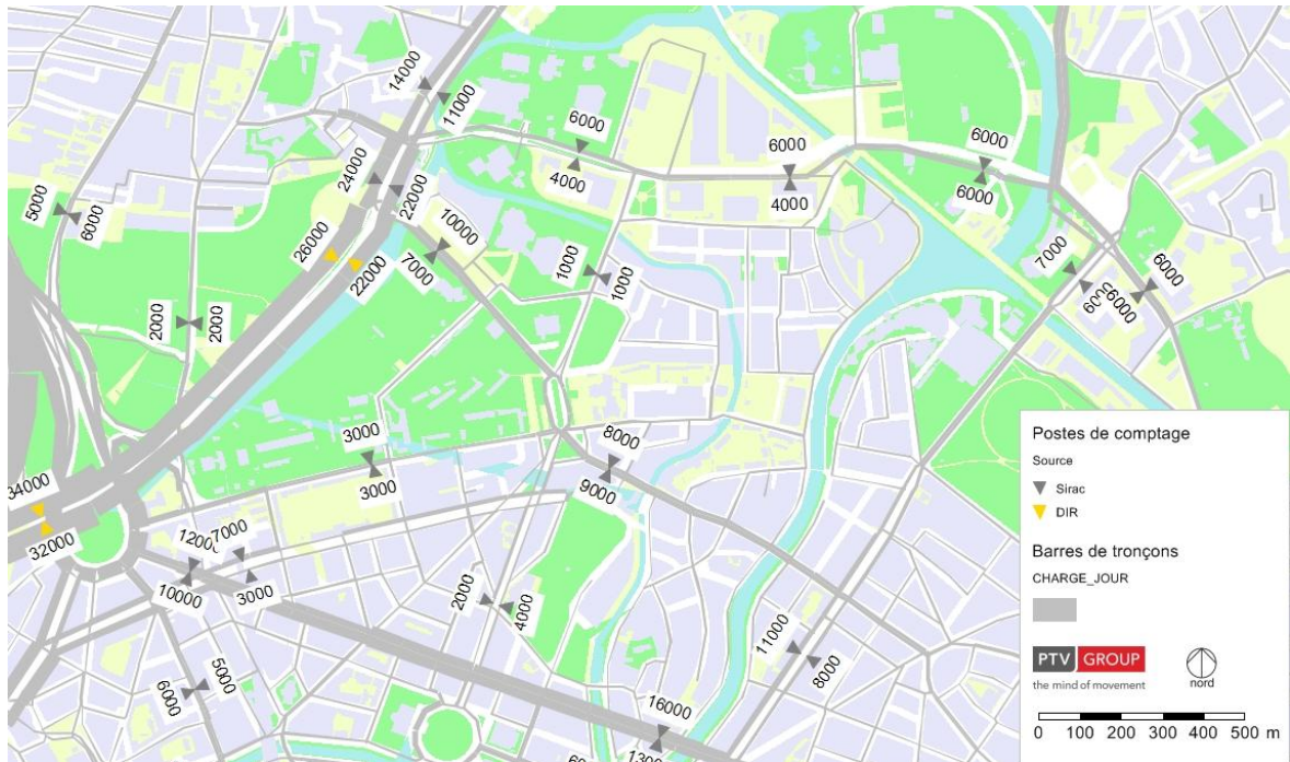
Fig. 1 : Le périmètre d'étude, charges journalières (TMJO) – ici mardis-judis de mars et octobre 2011
