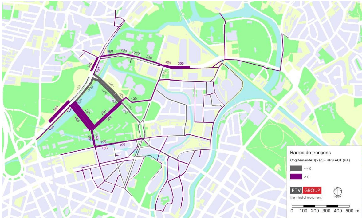
Fig. 47 : Effet nouveaux flux et nouveau barreau, HPS
