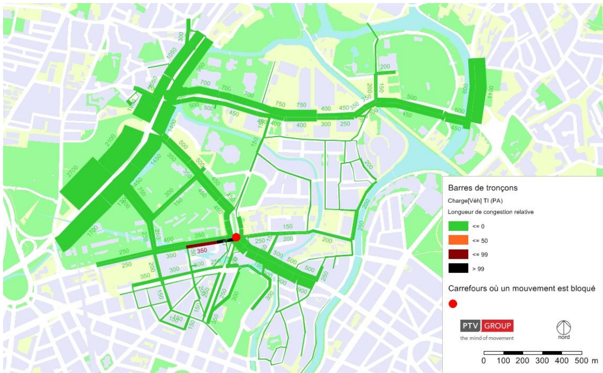
Fig. 54 : Photo des retenues à la fin de l'heure, moyen terme, nouveau barreau, sans Strauss, HPS
