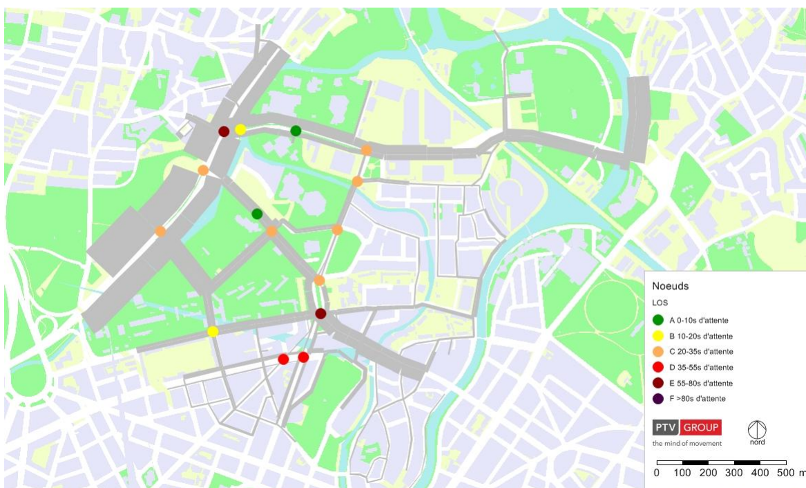
Fig. 28 : Temps d'attente moyens aux carrefours, long terme, nouveau barreau – Wenger Valentin - feux, HPS
