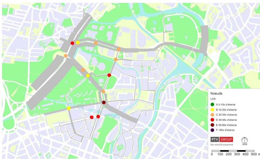
Fig. 36 : Temps d'attente moyens aux carrefours, moyen terme, réseau actuel, HPM
