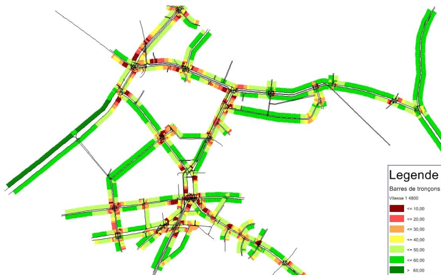
Fig. 60 : Vitesses moyennes sur une heure, situation actuelle, HPM
