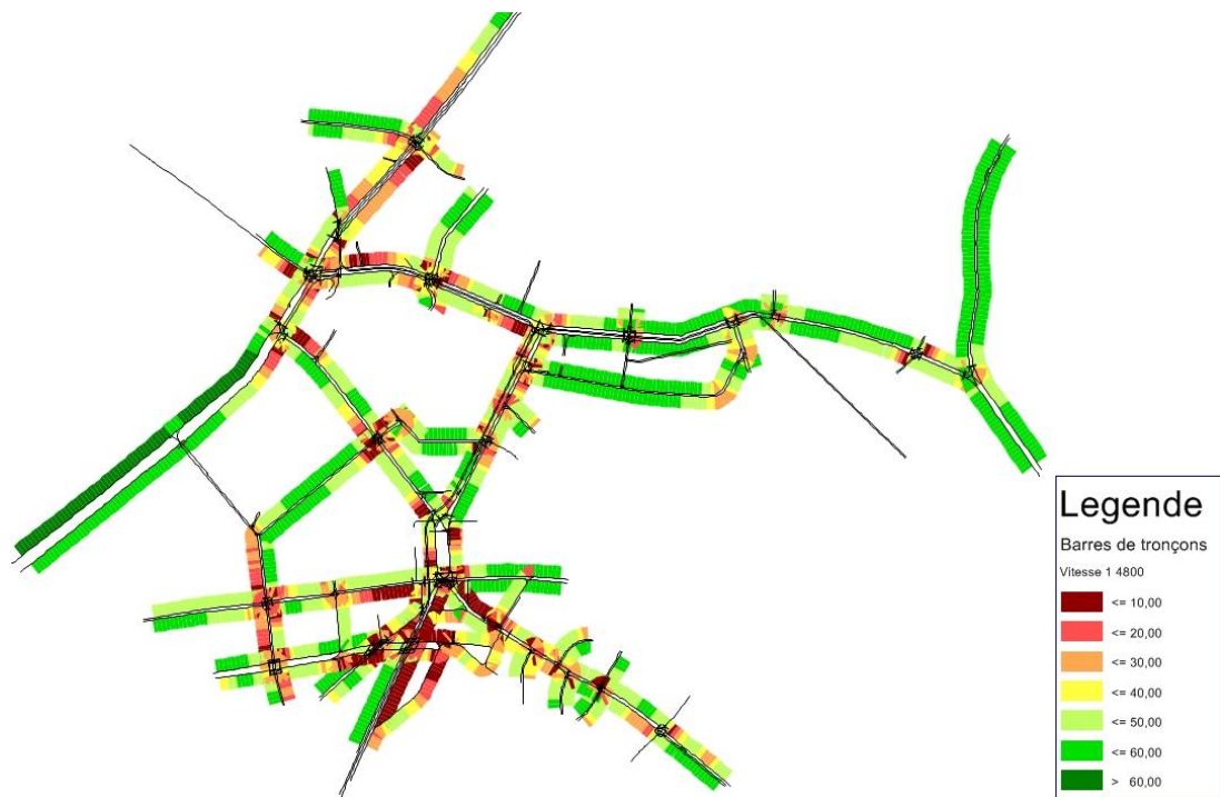
Fig. 62 : Vitesses moyennes sur une heure, situation actuelle, HPS
