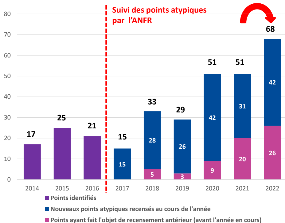
Nombre total de points atypiques par année
