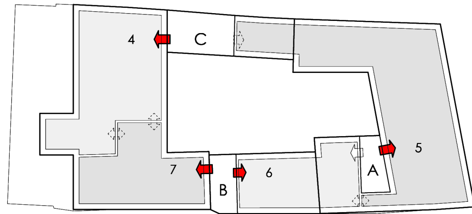
Etage 2 335,25 m 2 + (ABC)
