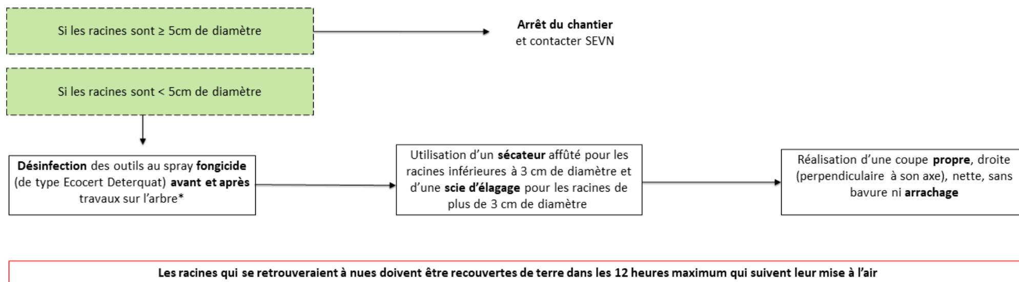
FIGURE 15 : SCHÉMA RÉCAPITULATIF DE LA MÉTHODOLOGIE À RESPECTER POUR LA COUPE DES RACINES
