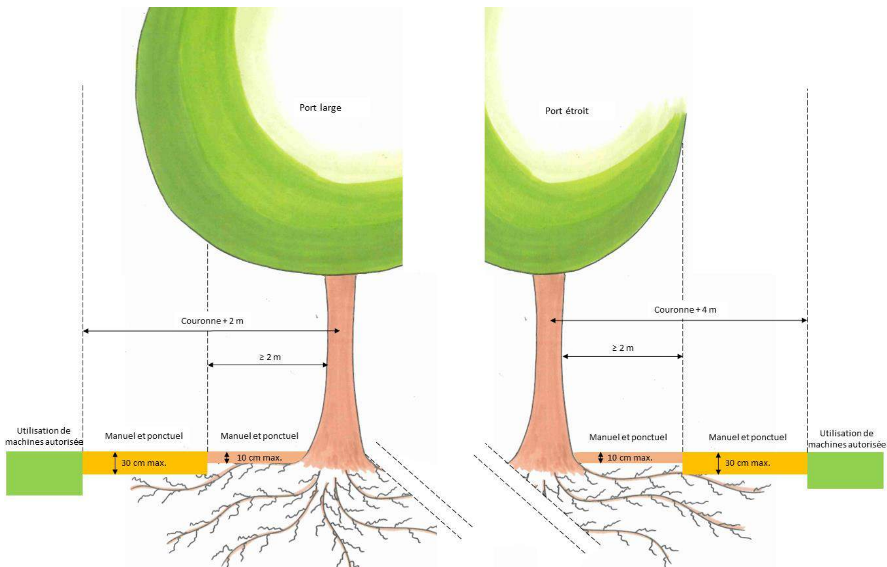
FIGURE 12 : SCHÉMA RÉCAPITULATIF DES PLANTATIONS POSSIBLES DANS ET AUX ABORDS DE LA ZONE PROTÉGÉE DE L'ARBRE EN ESPACE VERT
