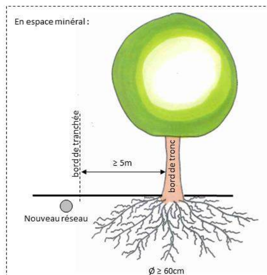
FIGURE 17 : SCHÉMA D'IMPLANTATION D'UN NOUVEAU RÉSEAU EN ESPACE MINÉRAL À PROXIMITÉ D'UN ARBRE EXISTANT D'UN DIAMÈTRE \geq 60 CM
