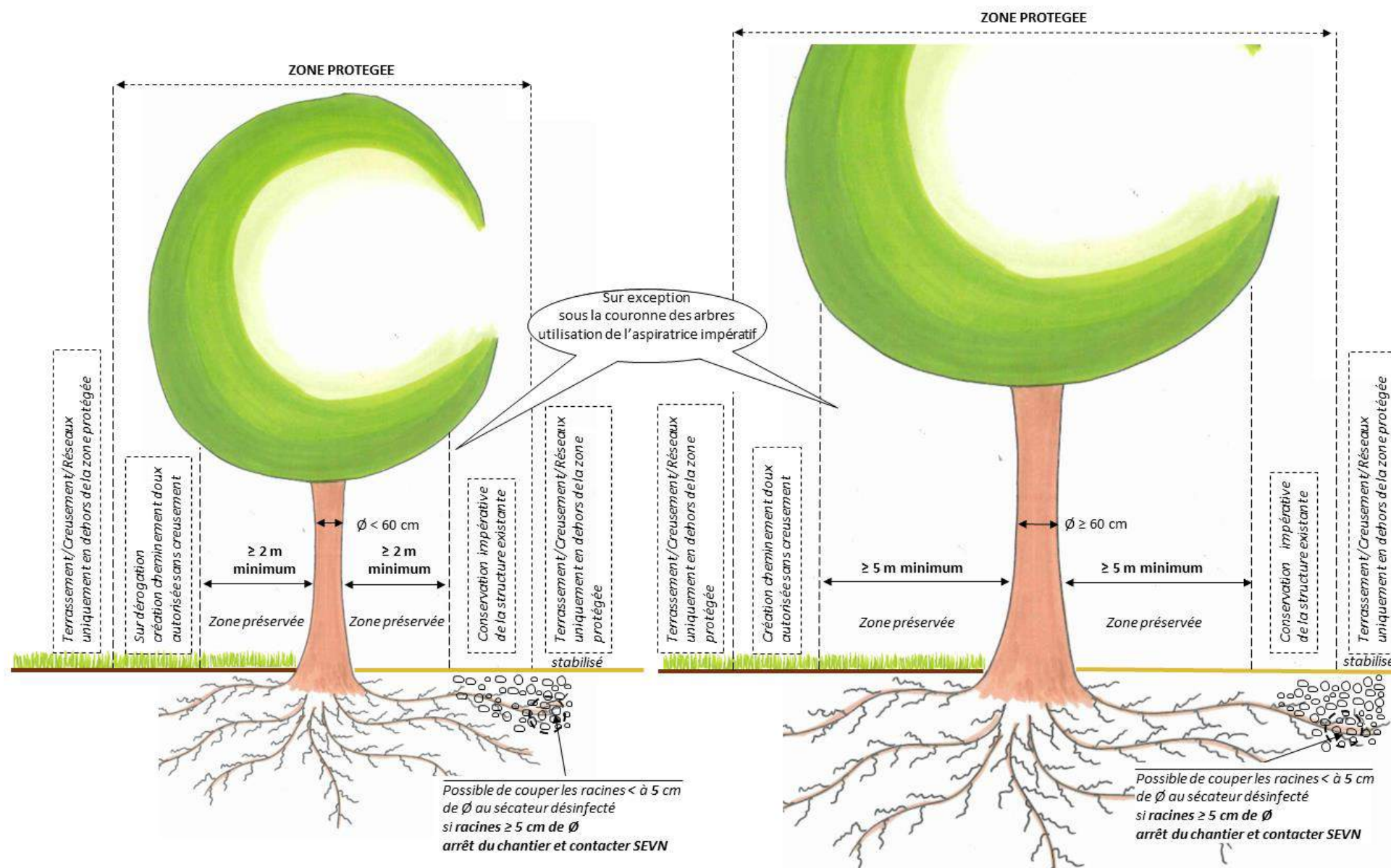
FIGURE 11 : SCHÉMA RÉCAPITULATIF DES INTERVENTIONS DE TERRASSEMENT DANS ET AUX ABORDS DE LA ZONE PROTÉGÉE DE L'ARBRE EN ESPACE VERT
