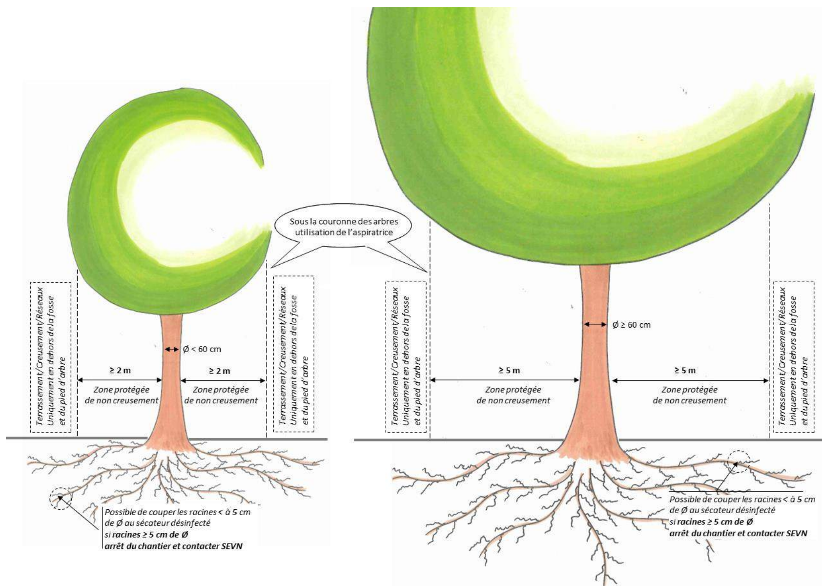
FIGURE 14 : SCHÉMA DES RÈGLES DE TERRASSEMENT/CREUSEMENT EN ESPACE MINÉRAL
